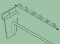
GANCIO SEMPLICE HOOK D. 6 mm
