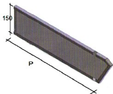
Fascia laterale SX cielino inclinato
